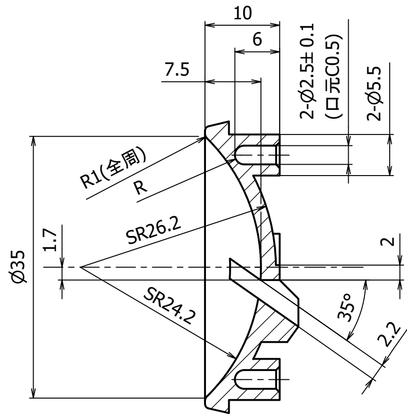
A-A (2:1)
